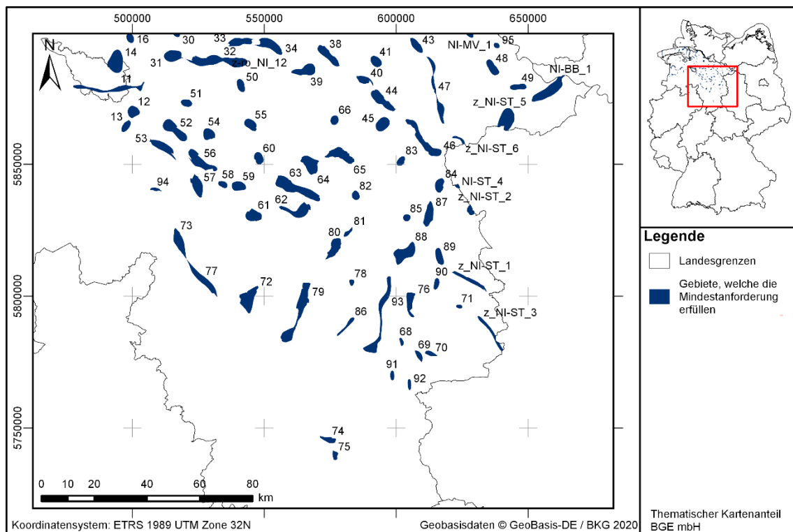
Abbildung 10: Überblick über den südlichen Teil des Modellierergebnis. Die Benennungen der Gebiete (abgebildet ohne „MG_d_“), welche die Mindestanforderungen erfüllen, ist Tabelle 14 zu entnehmen. Gebiet mit dem Präfix „MG_d_z_NI_“ sind nur mit der letztgenannten Nummer dargestellt.
