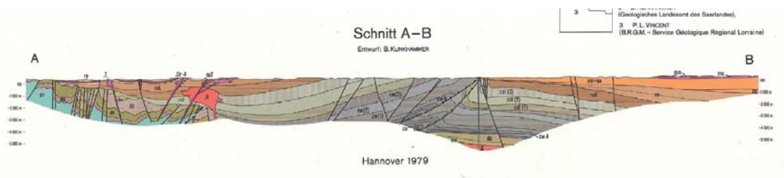
Abbildung 124 Schematischer geologischer Schnitt durch das Saar-Nahe-Becken (GÜK200 – CC 7102 Saarbrücken); Schnittlage Nordwest-Südost. Die Forschungsbohrung Saar 1 im Zentrum des Saar-Nahe-Beckens durchteuft Einheiten des Karbon und Devon und endet in Granit (in Rot dargestellt); Grundgebirge im NE des geologischen Schnitts sind devonische Einheiten (Tonschiefer, Sandsteine und Grauwacken).
