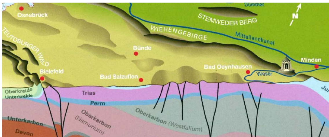
Abbildung 89: Vereinfachtes geologisches Profil durch das Norddeutsche Bergland/Wiehengebirgsvorland, modifiziert nach Schäfer (2016)
