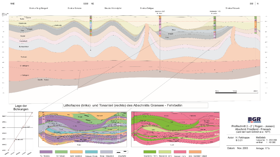
Abbildung 55: Profilschnitt von der Struktur Burg Stargard bis Struktur Friesack mit Lage der Bohrungen (Feldrappe 2003). Der Nordost-Südwest verlaufende Abschnitt bildet das Deckgebirge in den ausgewiesenen Gebieten in Brandenburg ab.
