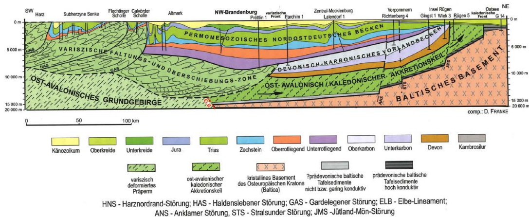
Abbildung 84: Geologisch-tektonischer Schnitt vom Harzvariszikum über Brandenburg bis zur Offshore-Bohrung G 14/1 in der südlichen Ostsee (Franke et al. 2015a)
